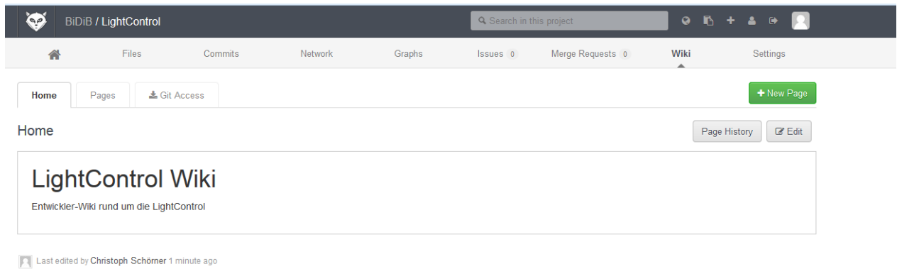
Abbildung 32: Git Wiki
